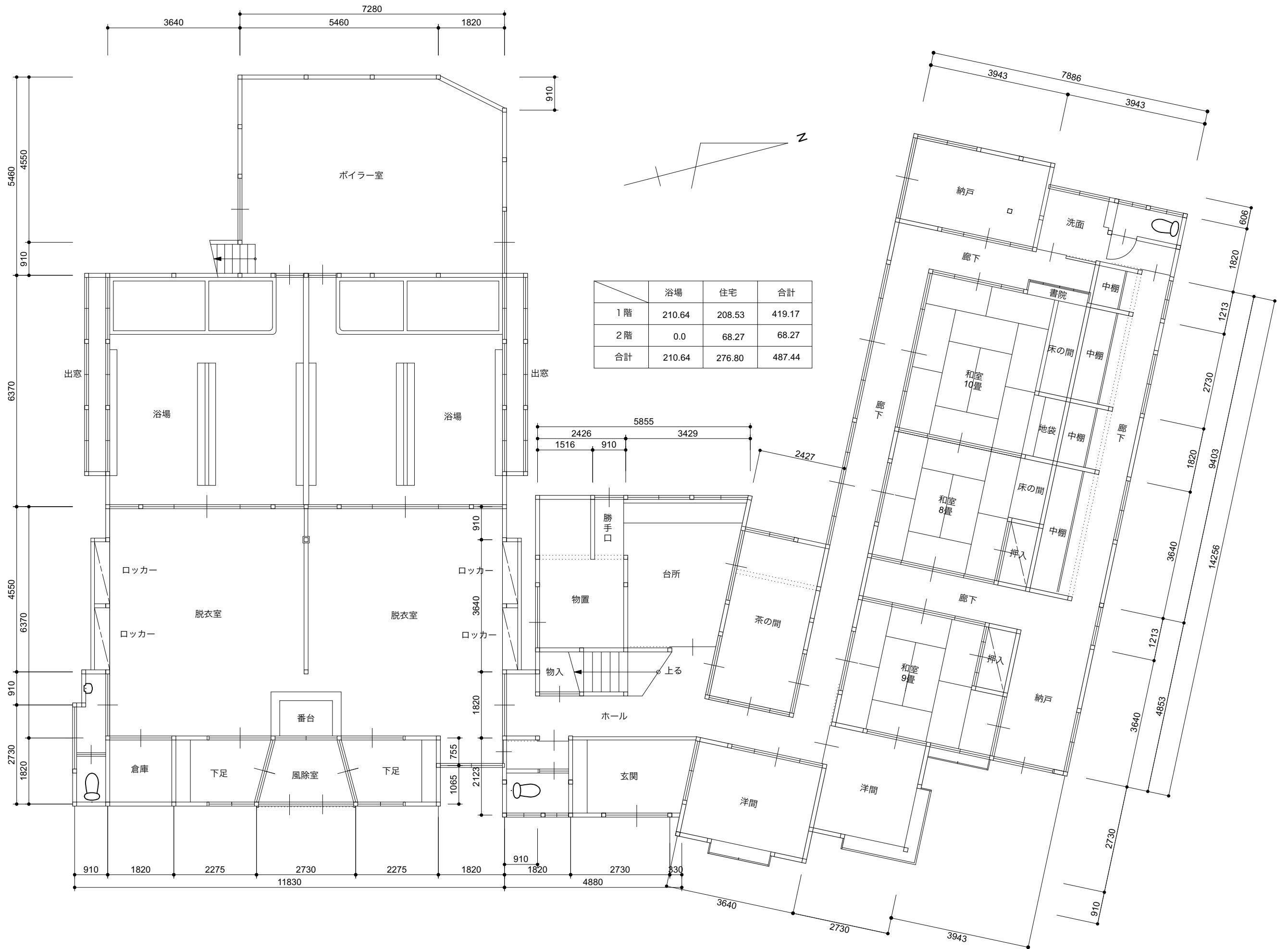
1階現況平面図 1:100
